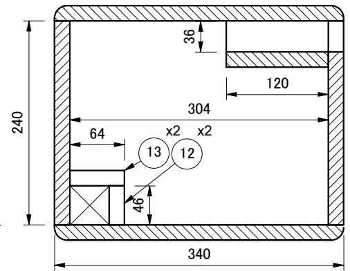
SECTION "GG"
